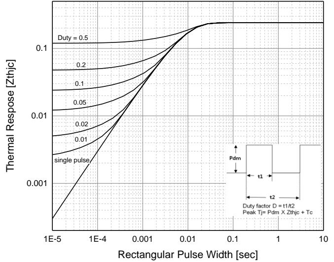
Fig. 14 Transient Thermal Impedance
