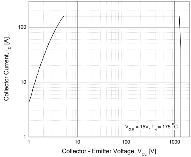
Fig. 18 RBSOA
